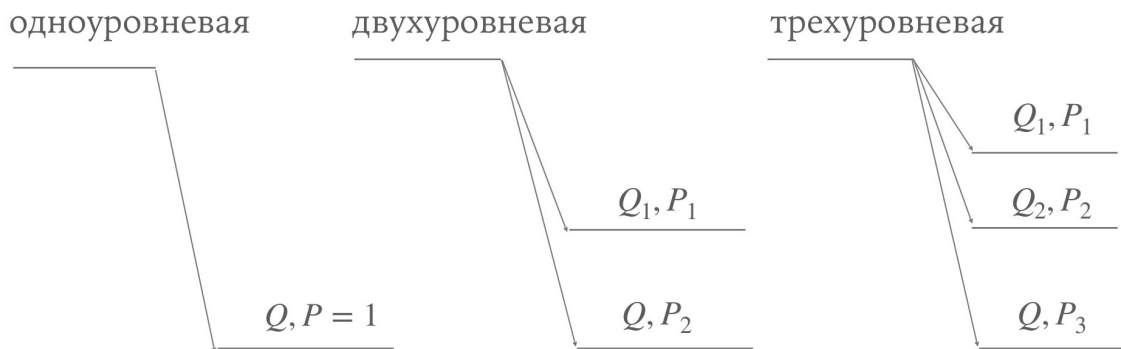
Рисунок 2.7 — Модельная схема распада дочернего ядра для ядер с неизвестными схемами распада.
