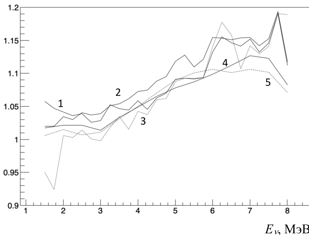
Рисунок 3.7 — Отношение спектра ^{235}\text{U} к сумме всех спектров с весами, соответствующими составу активной зоны во время измерения Double Chooz. 1 – Meuller [22], 2 – ILL [68; 69], 3 – Попов [51; 81], 4 – Vogel [63], 5 – МЕРФІ [65].
