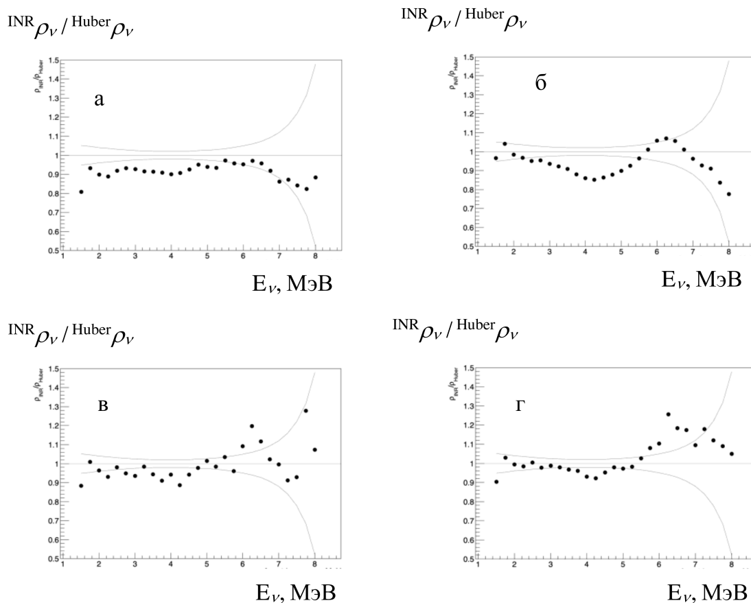
Рисунок 2.14 — Отношение спектров антинейтрино, полученных в данной работе, к спектрам из работ [22; 23] - черные точки: а – ^{235}\text{U} , б – ^{238}\text{U} , в – ^{239}\text{Pu} , г – ^{241}\text{Pu} . Показана оцененная погрешность расчетных спектров - сплошные кривые сверху и снизу.
