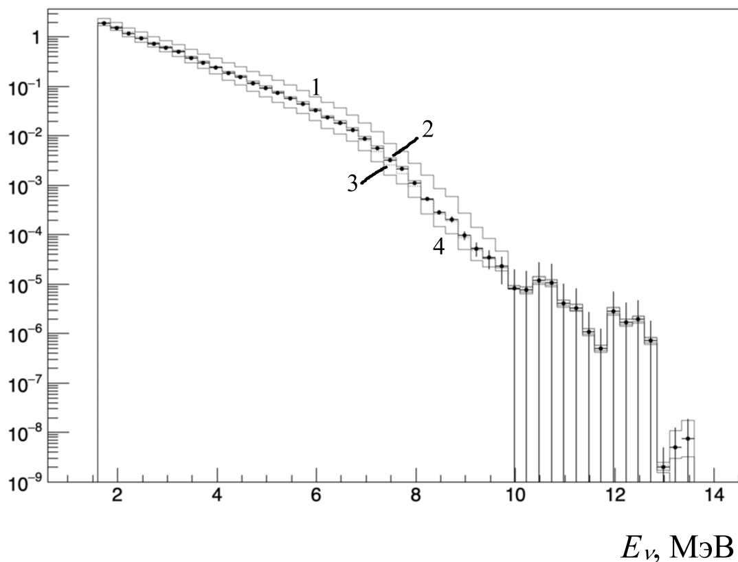
Рисунок 3.8 — Экспериментальные спектры антинейтрино делящихся изотопов ^{235}\text{U} , ^{238}\text{U} , ^{239}\text{Pu} и ^{241}\text{Pu} , полученные путем разделения экспериментального спектра Double Chooz (3.2). 1 — ^{238}\text{U} , 2 — ^{235}\text{U} , 3 — ^{241}\text{Pu} , 4 — ^{239}\text{Pu} . Черные точки с ошибкой — спектр Double Chooz.
